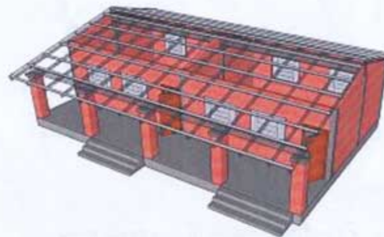
Axonometrías
